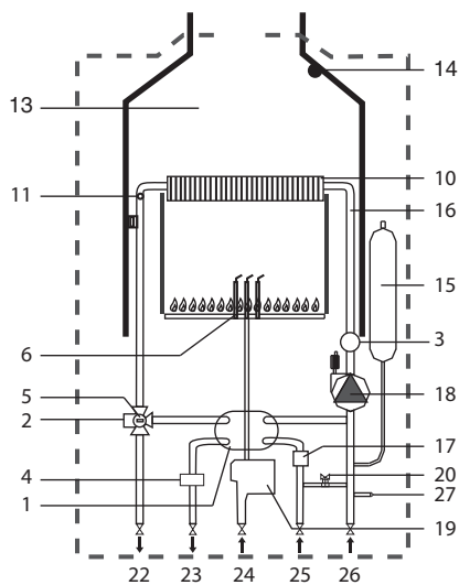
Принципиальная схема
