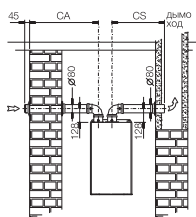
Воздухозабор через стену, дымоудаление в дымоход
