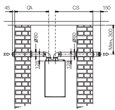
Воздухозабор и дымоудаление через стену
