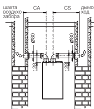
Воздухозабор из вентиляционной шахты, дымоудаление в дымоход
