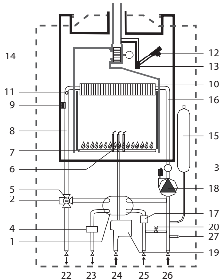
Принципиальная схема
