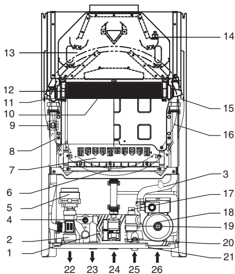
Внутренняя структура
