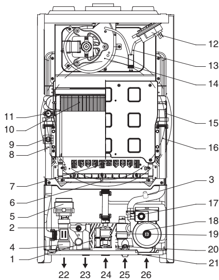
Внутренняя структура
